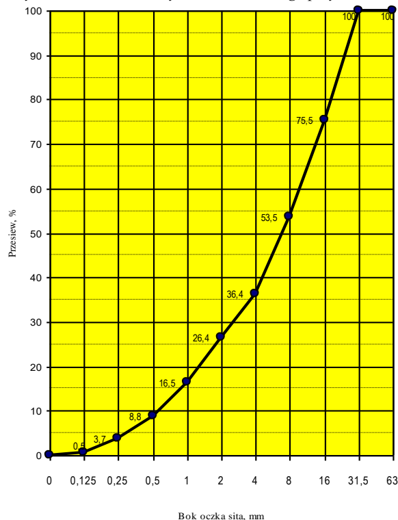
Rys. 1. Krzywa uziarnienia kruszywa do omawianego przykładu.
