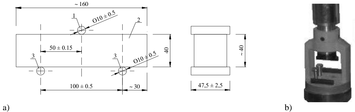
Rys.6.1. a) Schemat układu łamiącego do badania wytrzymałości na zginanie cementu: 1 - wałek obciążający; 2 - próbka; 3 - podpory b) Przystawka do zginania beleczek 40x40x160mm, zgodna z PN-EN 196
